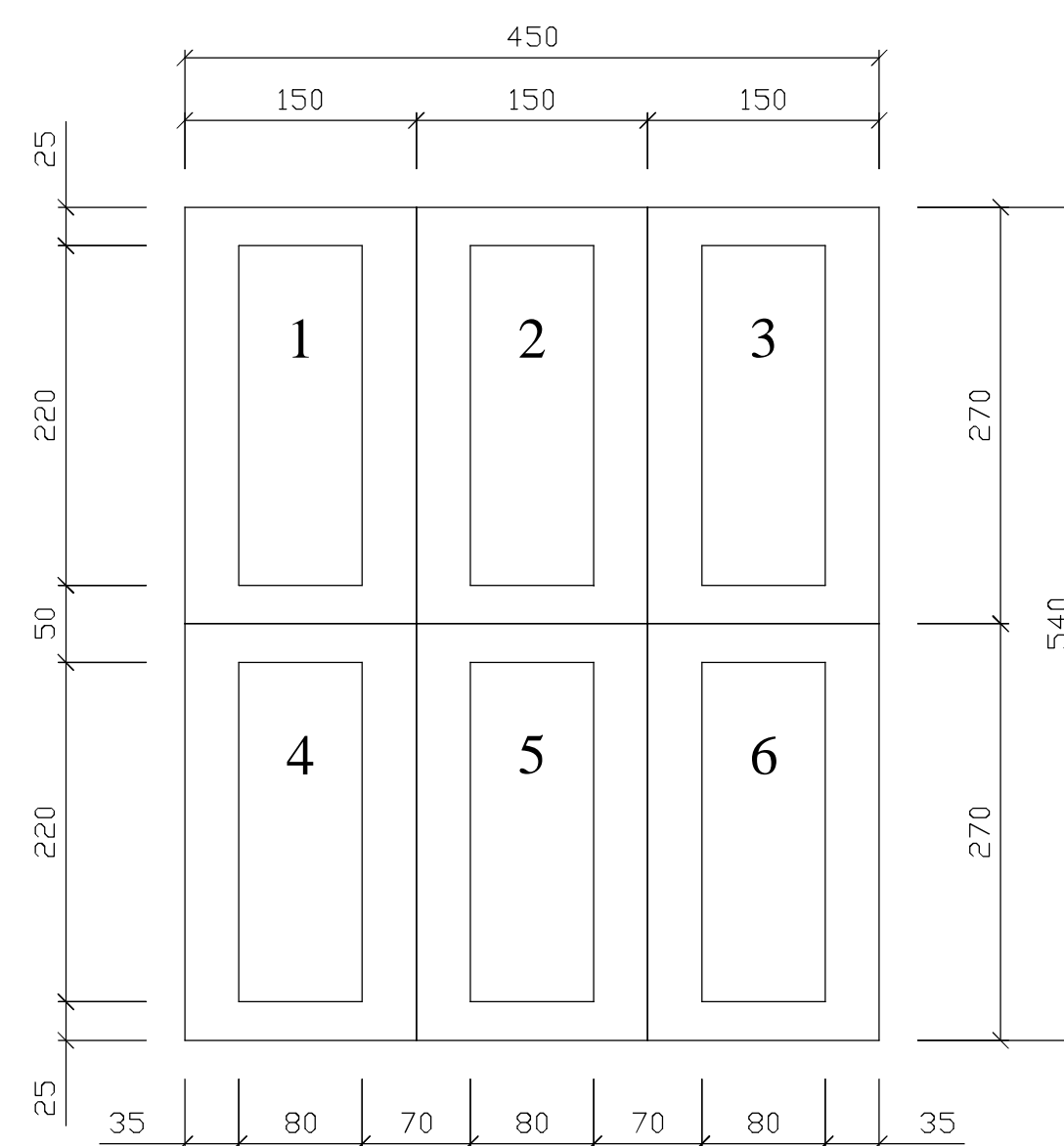
GRIGLIATO - FOSSE
