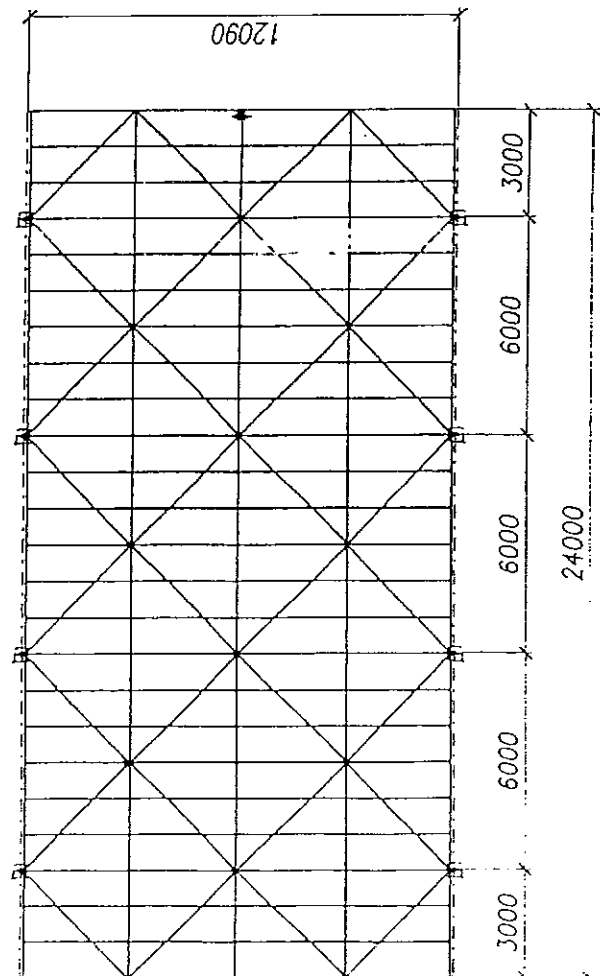
PIANTA
